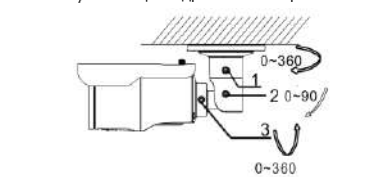
Рисунок 1-7 Настройка угла наблюдения камеры
